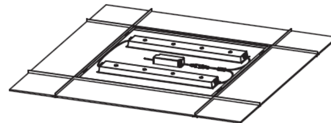
C: Fixez le filin de sécurité et installez le luminaire dans le plafond. D: Ajustez la position du luminaire et nettoyez-le.
